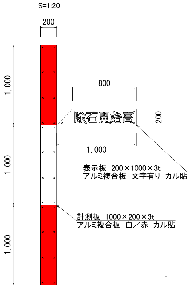
堆砂計測板 仕様図
