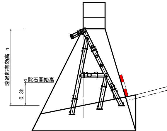
堆砂計測板 設置図(参考)
