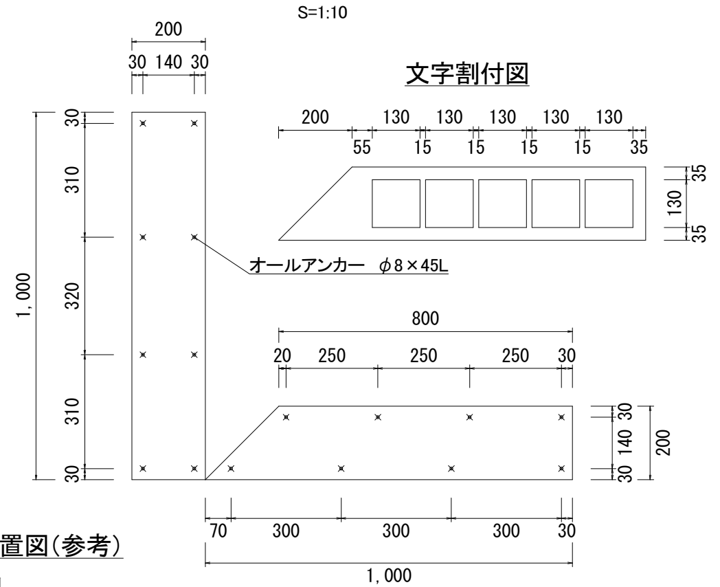
アンカー割付図
